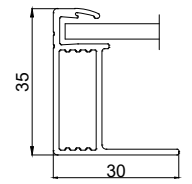
A-A 10: 1
